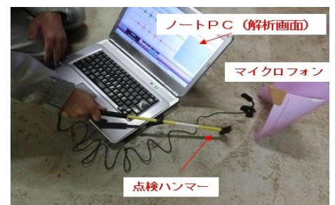
写真-2 マイクロフォンによる集録状況
